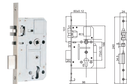
Optional mortise 6#
