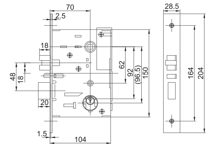
ANSI Mortise
